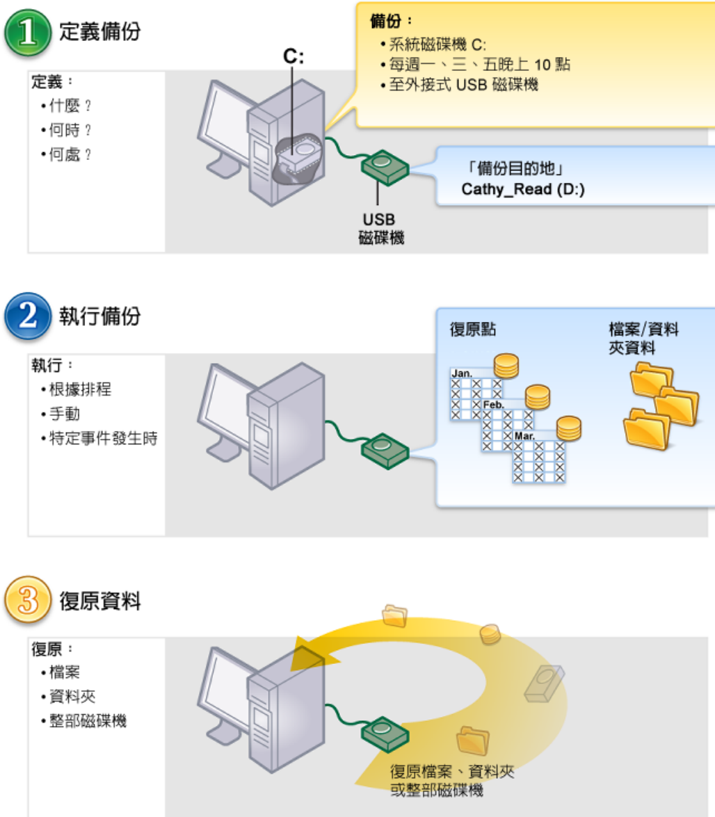
圖 4-1 使用 Symantec System Recovery
