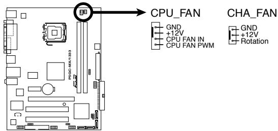
P5GC-MX/1333 Fan Connectors
