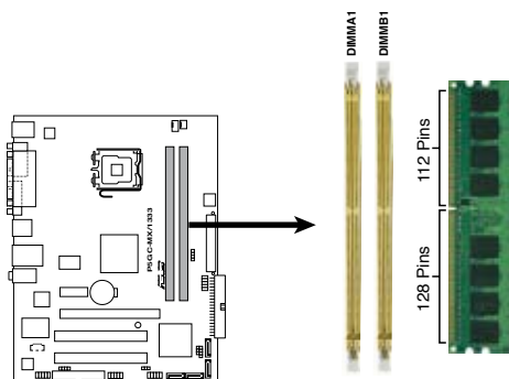
P5GC-MX/1333 240-pin DDR2 DIMM Sockets
