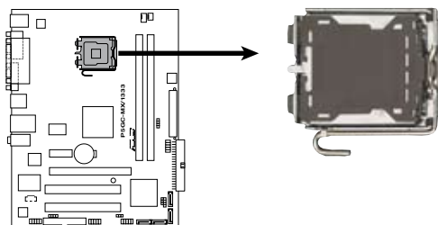
P5GC-MX/1333 CPU Socket 775
