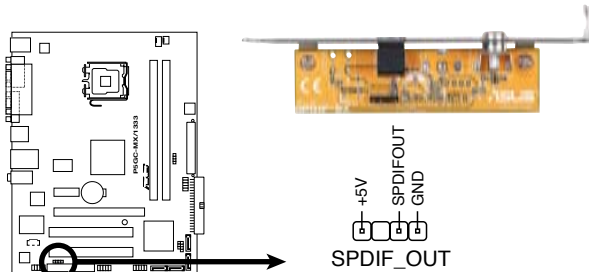
P5GC-MX/1333 Digital Audio Connector
