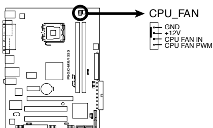
P5GC-MX/1333 CPU Fan Connector
